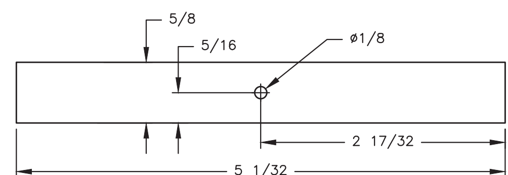
W-932DG DRILL GUIDE FULL SCALE
