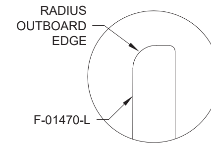
FIGURE 3: SIDE SKIN EDGE RADIUS
