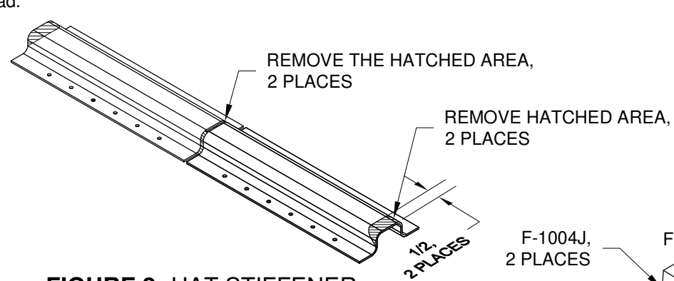
FIGURE 2: HAT STIFFENER
